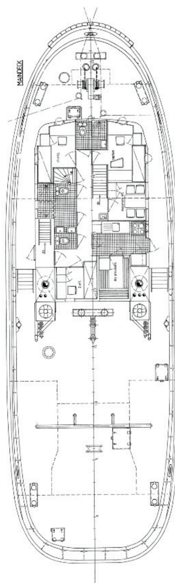
TWEEN DECK
